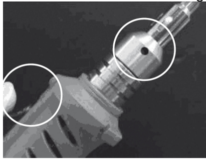
Blaue Flamme in der Bohrung
